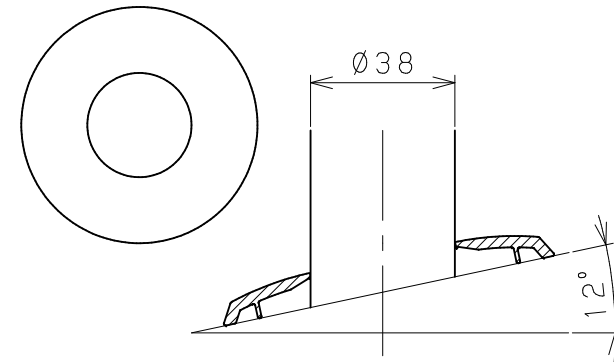
勾配12° (カット不要) 1:2
